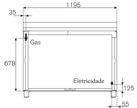
VISTA TRASEIRA
